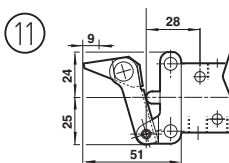
Impieghi pesanti - unidirezionale - G1/8 valvole
