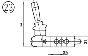
Valvola con azionamento a leva e ritorno a molla – G1/8 valvole
