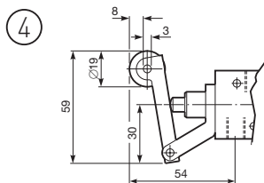
Leva-rotella - G1/8 valvole
