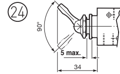
Interruttore – G1/8 valvole
