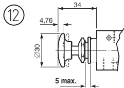
Pulsante – G1/8 valvole
