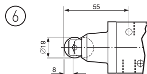
Rotella - G1/4 valvole
