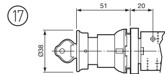
Pulsante/chiave – G1/8 valvole
