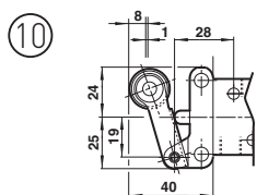
Leva-rotella per servizio pesante - G1/8 valvole
