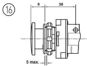
Stop di emergenza– G1/8 valvole
