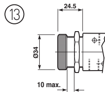
Pulsante (protetto) – G1/8 valvole
