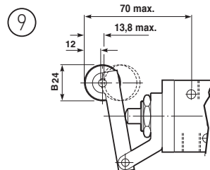
Leva-rotella - G1/4 valvole
