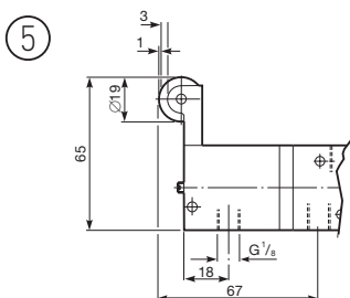
Leva-rotella sensibile - G1/8 valvole
