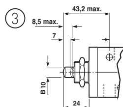
Pulsante - G1/4 valvole
