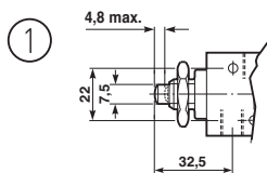
Pulsante - G1/8 valvole
