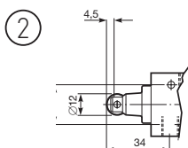
Rotella - G1/8 valvole
