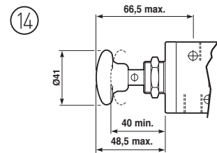
Pulsante – G1/4 valvole
