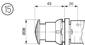
Pulsante (palmere)– G1/8 valvole
