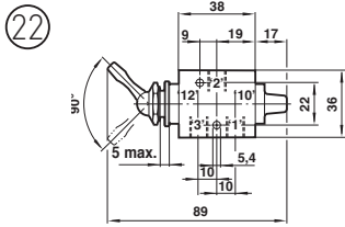
Valvola con azionamento a leva e ritorno a molla – G1/8 valvole
