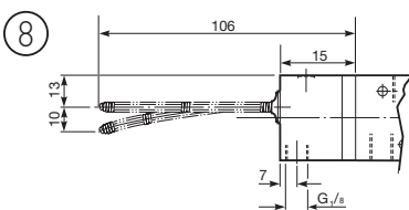
Baffo - G1/8 valvole
