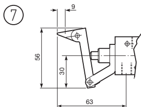
Unidirezionale - G1/8 valvole
