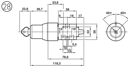
chiave – G1/8 valvole
