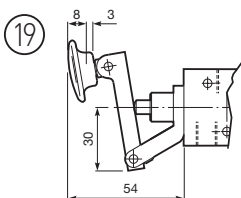
Leva/manopola – G1/8 valvole
